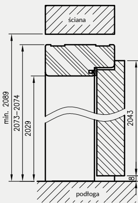
Przekrój pionowy OP do drzwi przylgowych
