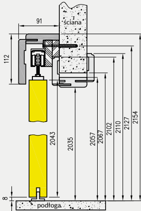
NT - przekrój pionowy na tunelu z ką. 63 mm
