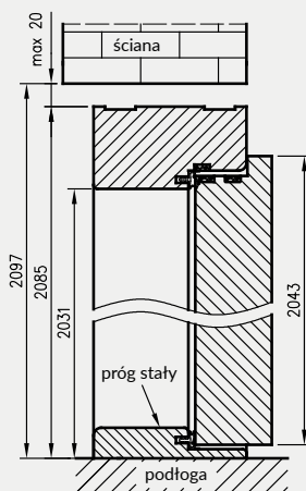
Ościeżnica drewniana do drzwi Athos z progiem stałym
