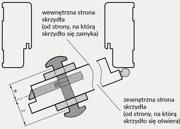
Rys. Dobór wymiaru wkładki z gałką
