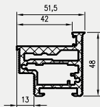
Profil do drzwi bezprzylgowych otwieranych na zewnątrz
