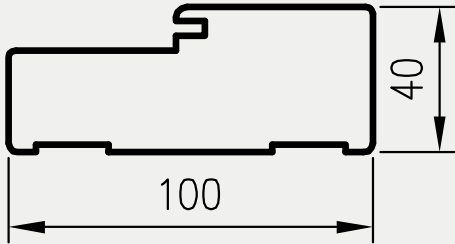
Profil OPB
