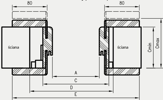
B-B Przekrój poziomy
