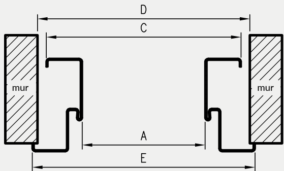
Wymiary szerokości OSS
