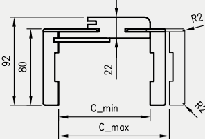
Przekrój ORB 095-300
