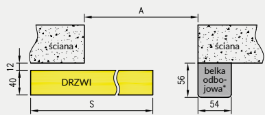
NS - przekrój poziomy (system lewy)
