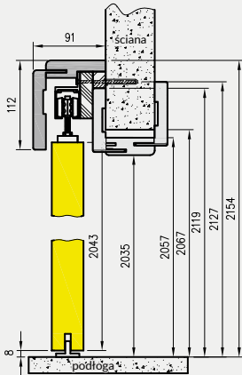
NT - przekrój pionowy na tunelu z ką. 80 mm
