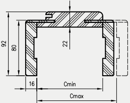
Przekrój poziomy OR/ORC
