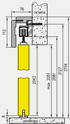
NS - przekrój pionowy
