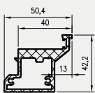
Profil DRE do drzwi przylgowych otwieranych do wewnątrz
