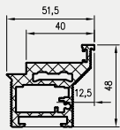
Profil do drzwi przylgowych otwieranych do wewnątrz
