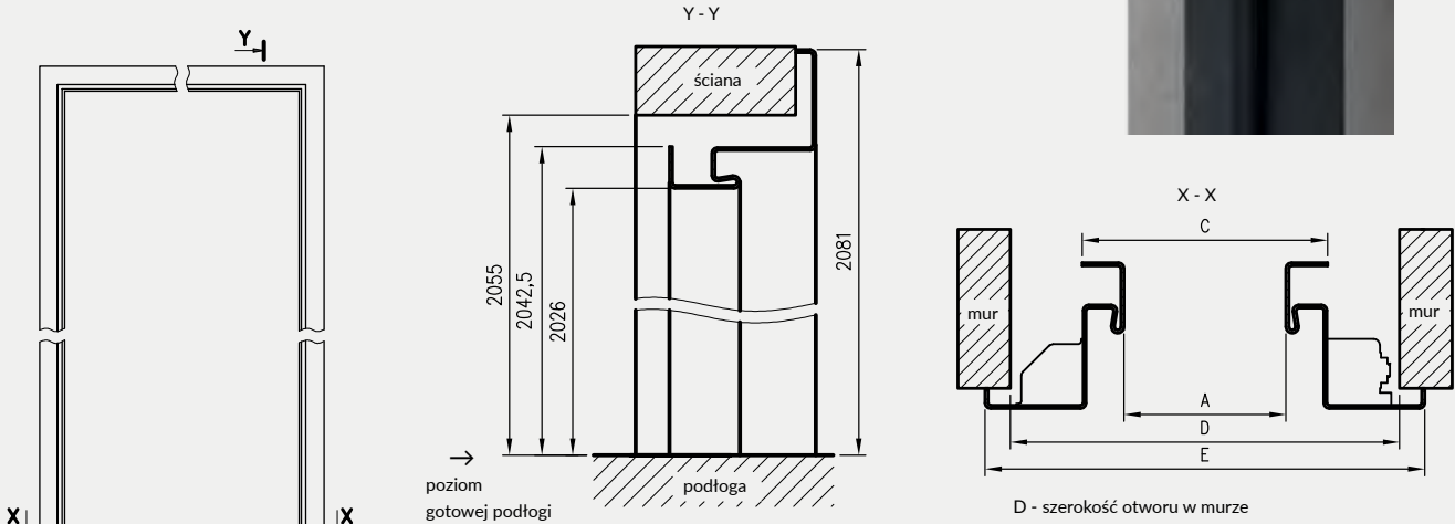
wymiary dla drzwi jednoskrzydłowych
