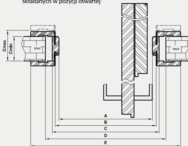
Przekrój poprzeczny drzwi składanych w pozycji otwartej*
